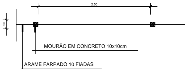
PLANTA DO DETALHE
