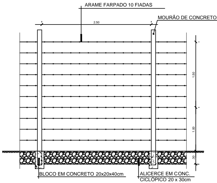
DETALHE DA CERCA DE MOURÃO
